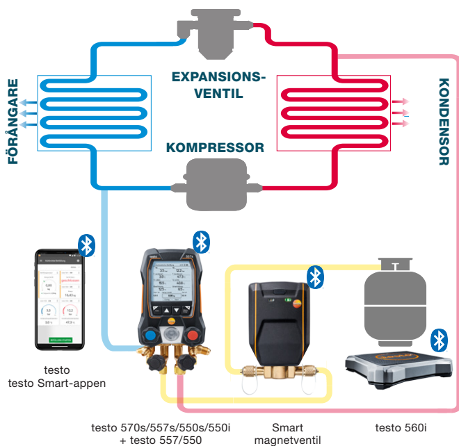
Schematiskt diagram för automatisk köldmediefyllning
