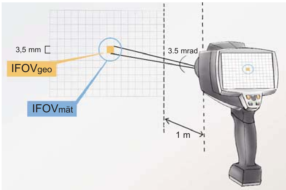
Bild 1.4: Synfält för en enskild pixel
