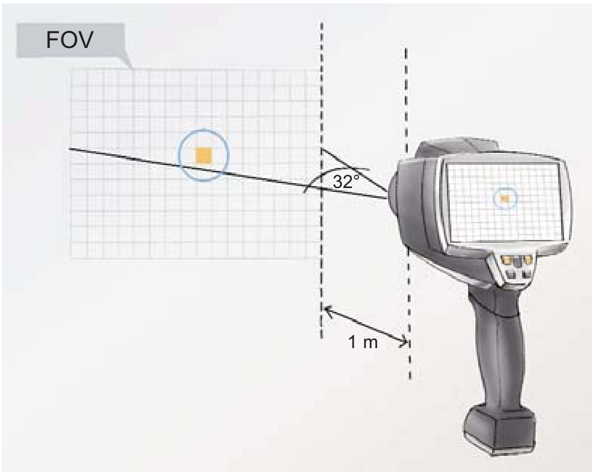
Bild 1.3: Värmekamerans synfält
