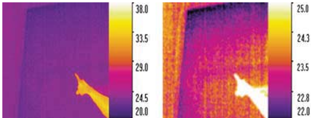
Bild 2.4: Justera temperaturskalan
