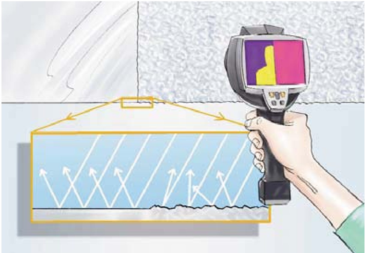
Bild 2.3: Speglande och diffus reflektion
